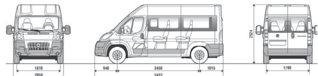
Panorama MH2 empattement 3450 mm
