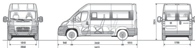
Combi MH2 empattement 3450 mm
