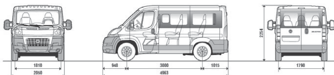
Panorama CH1 empattement 3000 mm
