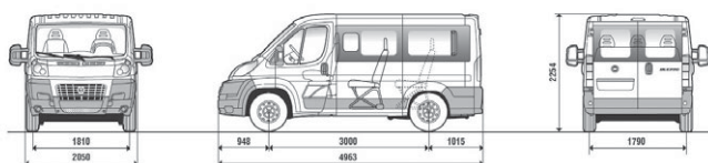
Combi CH1 empattement 3000 mm
